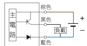
( PNP 輸出 )
