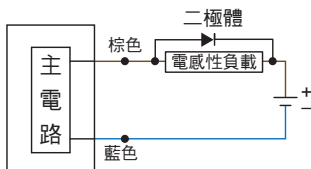
二線式類型
