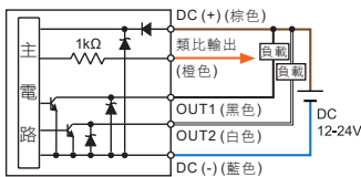
KP50E□ - 010 - □ 2NPN + 類比電壓輸出 (1 ~ 5 V)
