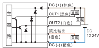
KP50E□ - 011 - □ 2NPN + 類比電流輸出 (4 ~ 20 mA)
