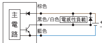
NPN類型
