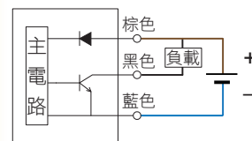
( NPN 輸出 )
