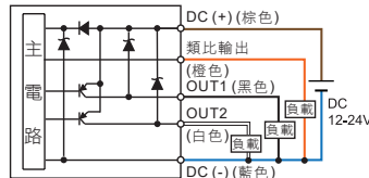
KP50E□ - 031 - □ 2PNP + 類比電流輸出 (4 ~ 20 mA)
