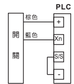
PLC輸入模組 (PNP)
