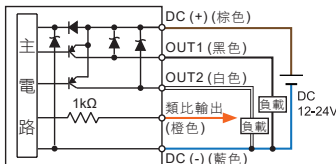
KP50E□ - 030 - □ 2PNP + 類比電壓輸出 (1 ~ 5 V)
