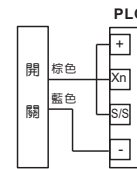
PLC輸入模組 (NPN)
